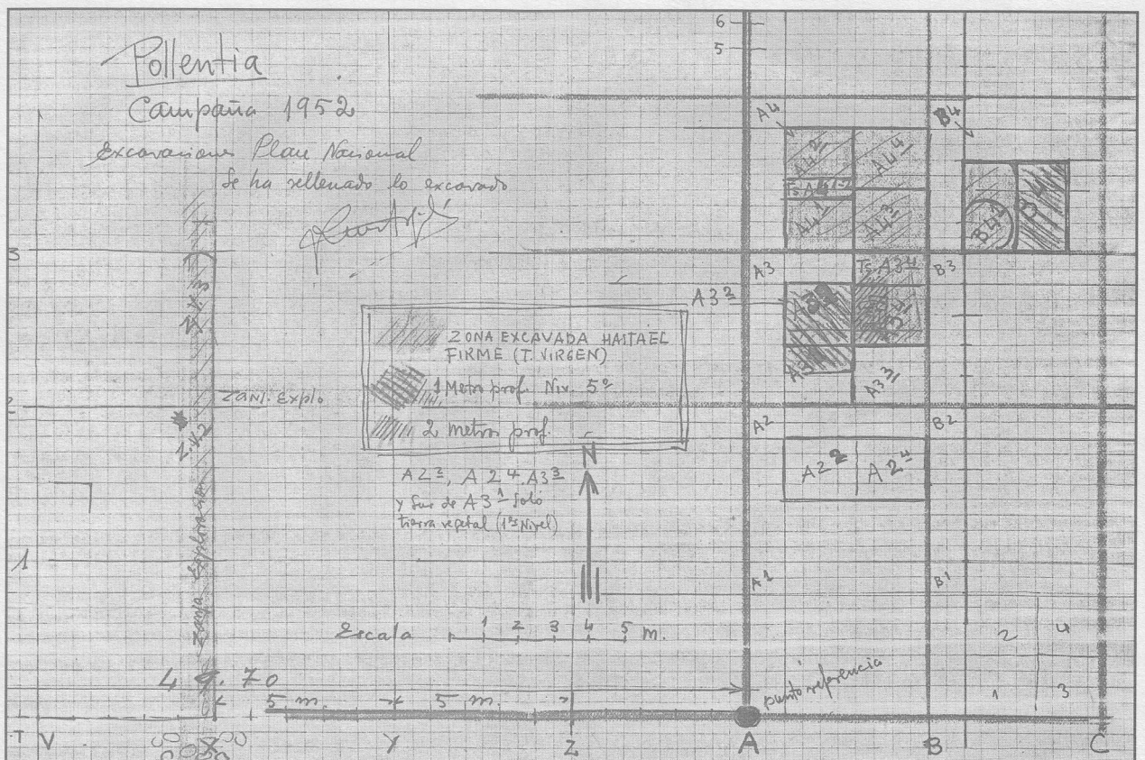
Plànol de les excavacions que Argilés i Ensenyat feren a l'est de l'oratori de Santa Anna l'any 1952.
