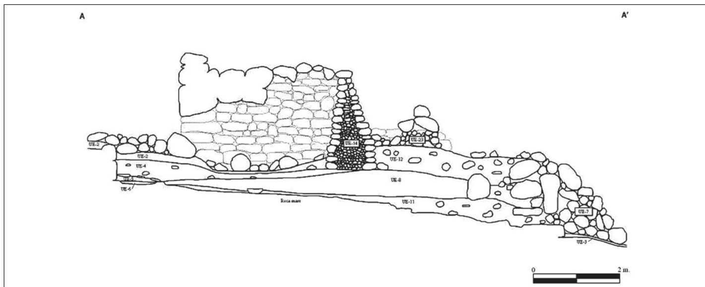
Secció longitudinal del passadís interior del talaïot est.
