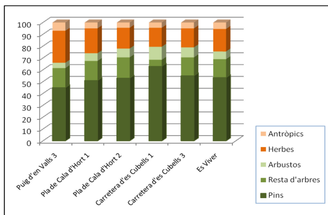
Figura 3.- Resultats de les anàlisis pol·líniques per grups representats.
