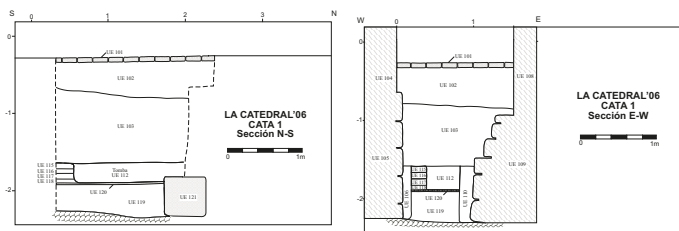
Figura 4: Secció de la cala 4
