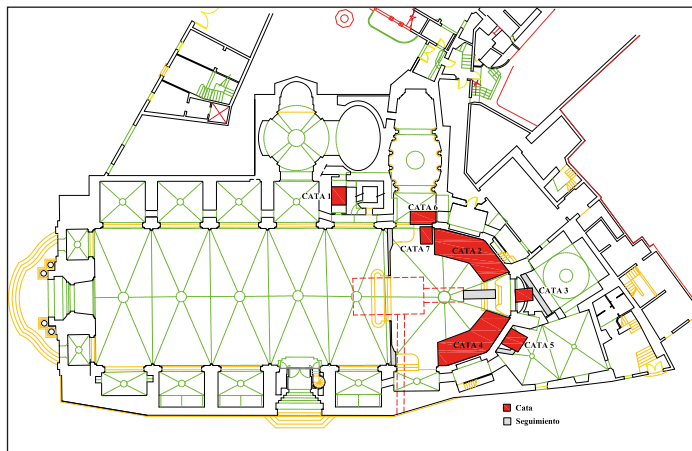
Figura 1: Planta general amb la situació de les cales i seguiments arqueològics
