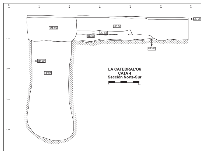
Figura 2: Seccions de la cala 1
