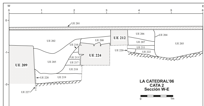
Figura 3. Secció longitudinal de la cala 2
