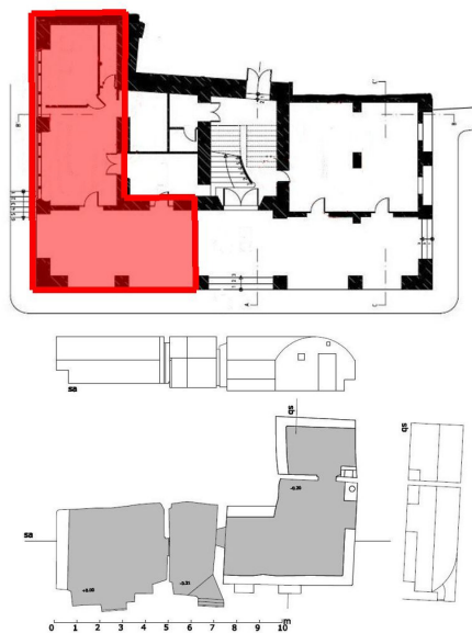
Figura 3. Ubicació de la presó respecte de l'edifici, a dalt; i planta de la presó, a baix.
