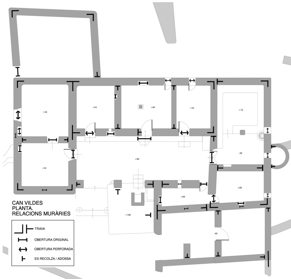
Figura 2. Plànol de relacions entre els murs de la casa pagesa coneguda com can Vildes, a Sant Antoni de Portmany, Eivissa. Estudi realitzat el 2007 per A. Ferrer.
