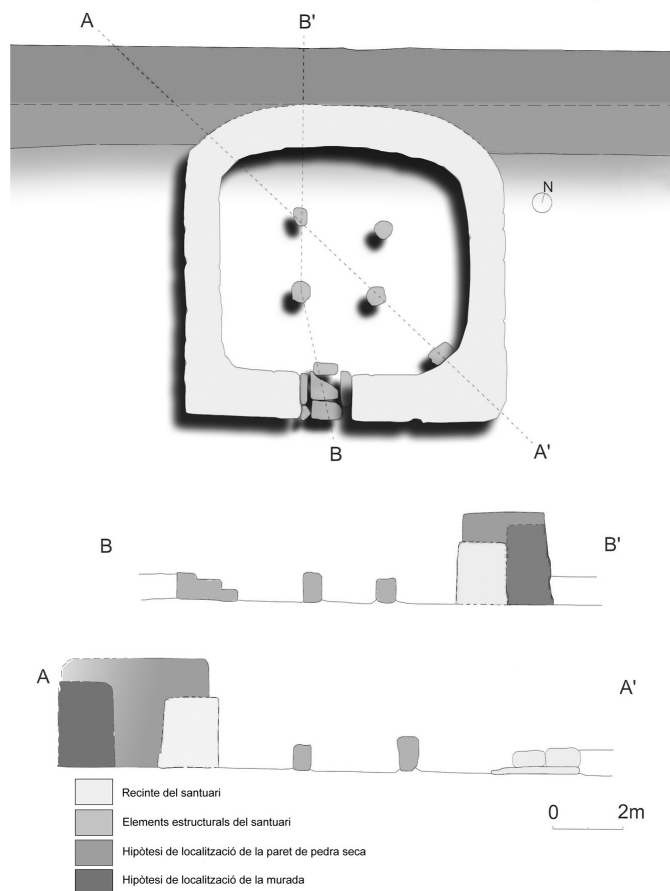
Fig. 2. Croquis de la planta i seccions del santuari segons Colominas (1923), modificada a partir de les interpretacions fetes en aquest treball. Les línies discontinues indiquen les hipòtesis sobre els límits de la façana posterior del recinte i de la murada.
