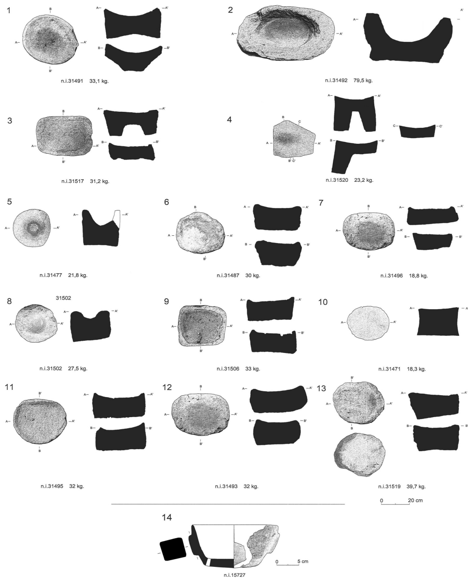
Fig. 4. Dibuixos zenitals i seccions dels macrolítics d'Els Antigors, conservats en el MAC.
