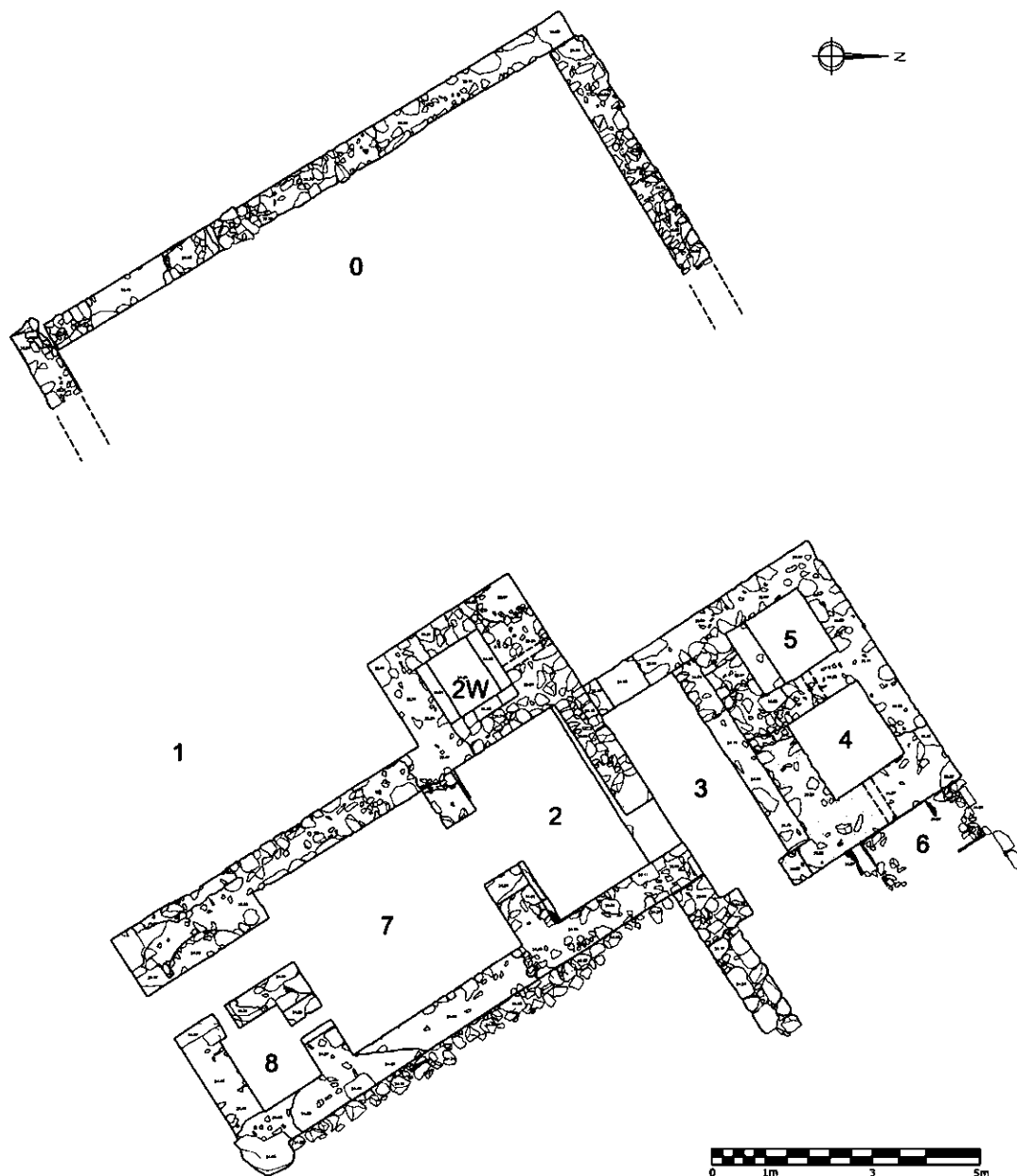
Figura 1. Planta de l'edifici termal de la vil·la romana de Son Sard. Els espais núm. 0, 1, 6 i 7 romanen sense excavar i corresponen hipotèticament a la palestra , un forn, un pati (latrines?) i al tepidarium , respectivament. Espais excavats: caldarium (2), praefurnium (2W), apodyterium (3), frigidarium (4 i 5) i laconium ? (8).
